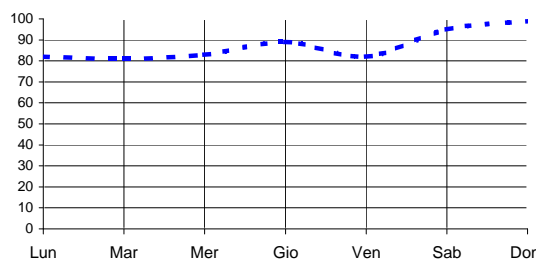
Umidità media -settimana dal 1/5/17 al 7/5/17
