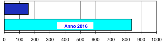
Temperatura media del terreno a 20 cm di profondità' - Mese Maggio 2017 e confronto con il 2016
