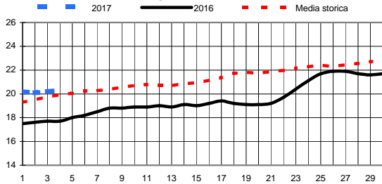
Temperatura media del terreno a 20 cm di profondità - Mese Giugno 2017 e confronto con il 2016
